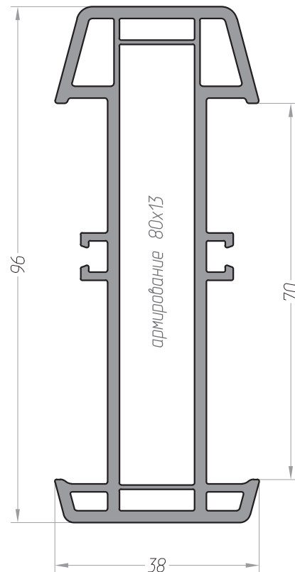
Профиль соединительный 38/70 арт. 10405038
